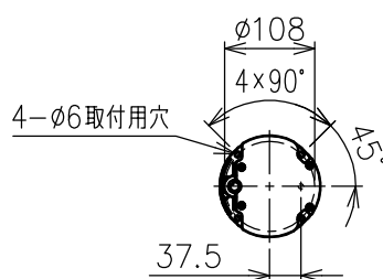
取付板詳細図
