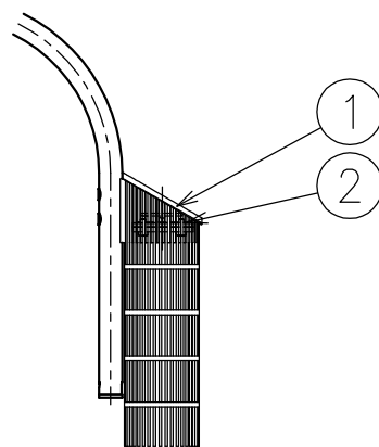
灯具詳細図 (S=1/5)
